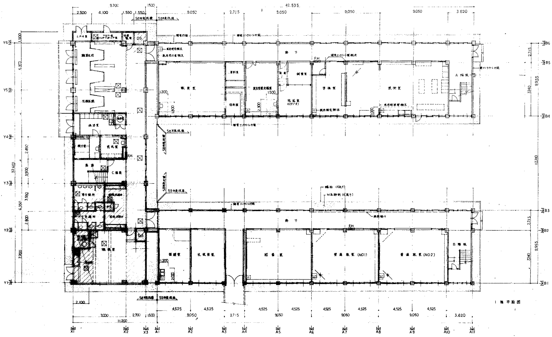
校舍 1階平面図
