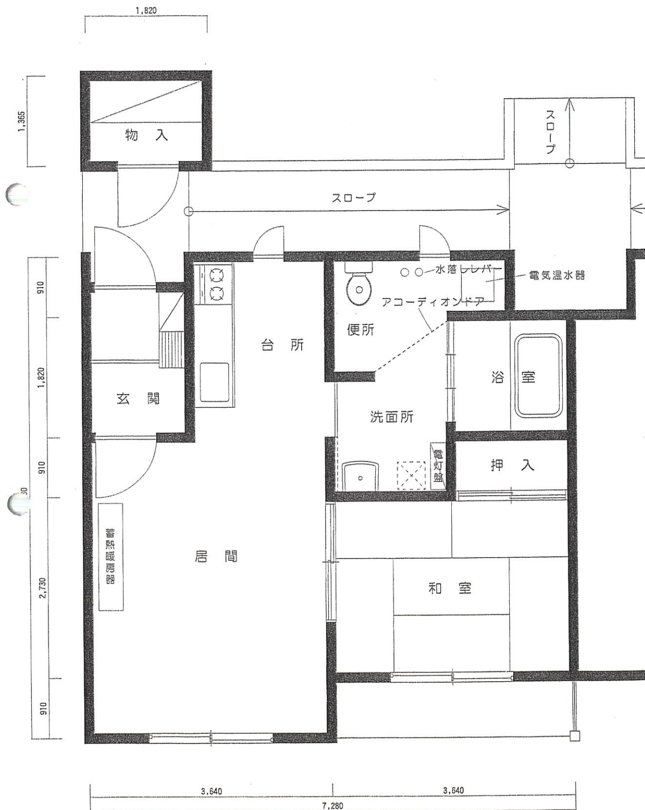
平面図 (1LDK) S=1/50
