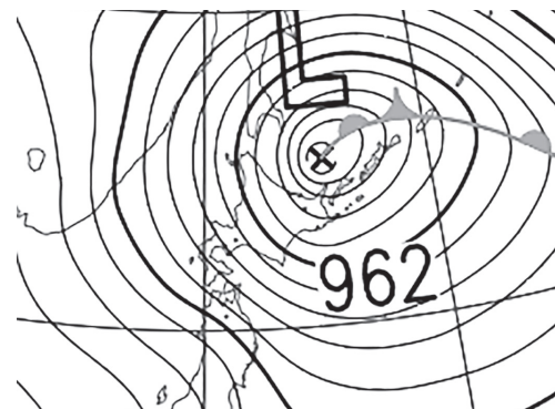
平成 30 年 3 月 2 日午前 9 時の地上天気図 (暴風雪により、道内各地で被害が発生)
